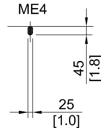
Fangbügel-Querschnitt Lifting hoop cross section
