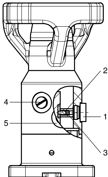
Einstellung Bedämpfungsnocke
